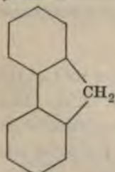
Fluorene.
